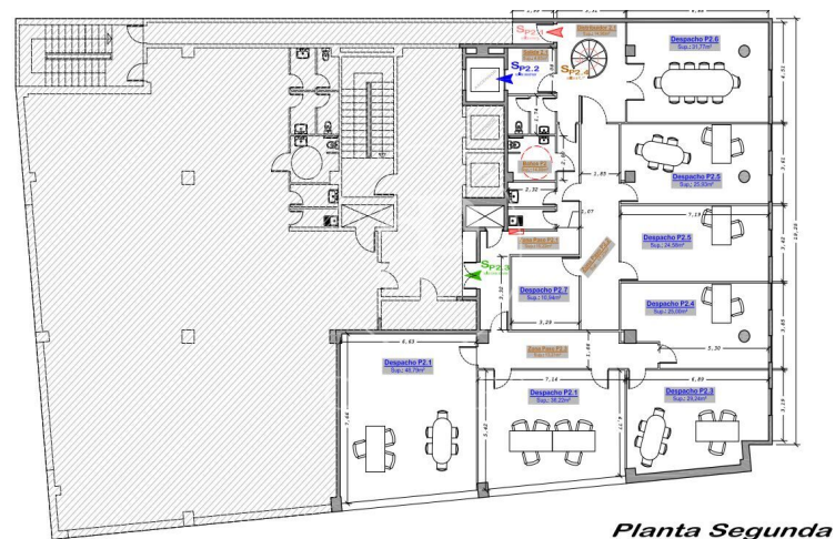
Planta Segunda
